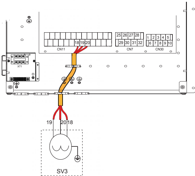
7.6.9 Trieigiui vožtuvui SV3
