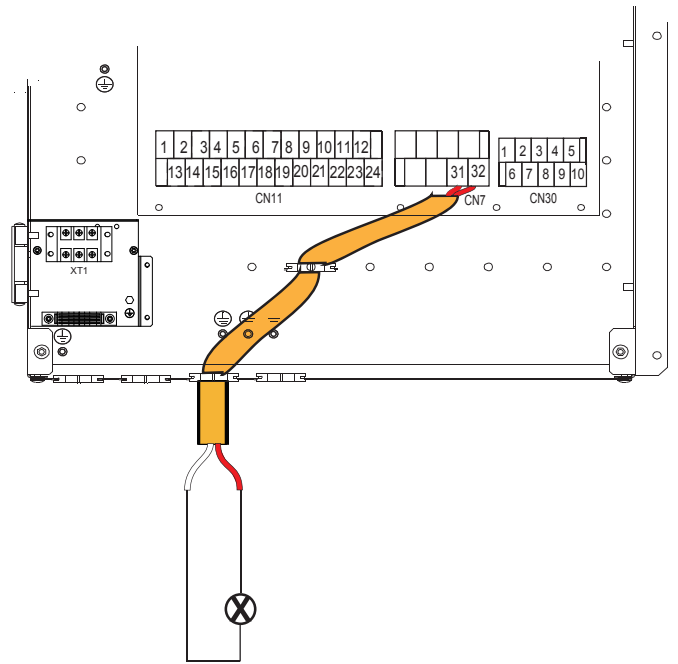
7.6.10 Atitirpinimo signalo išvesčiai
