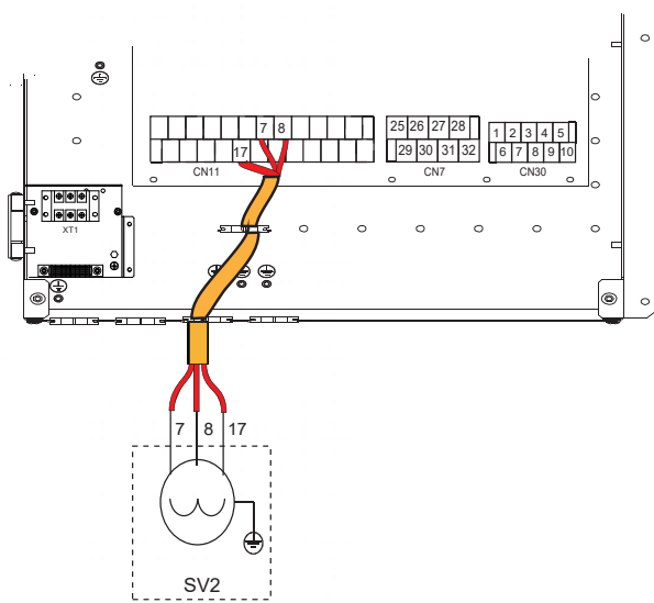
7.6.8 Trieigiui vožtuvui SV2
